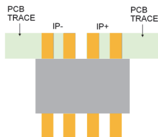
図15： Horizontal Portion Connection
