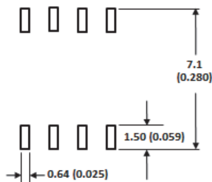
図12： Land Pattern for 4-mm Creepage
