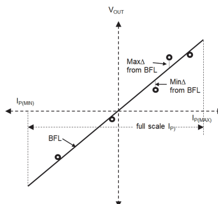
図11： Nonlinearity Calculation
