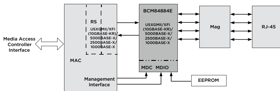
BCM84884E Block Diagram
